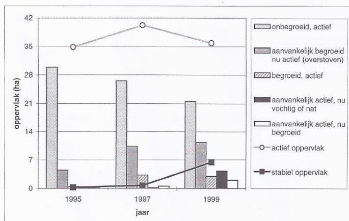
Figuur 8 • Oppervlakten van kaartenheden zoals weergegeven in.
