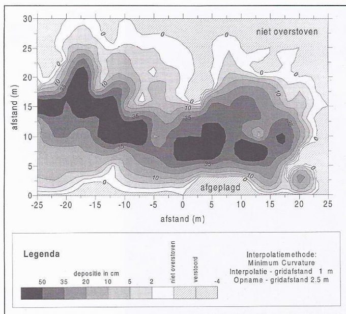
Figuur 4 • Overstuiving in struweel.
